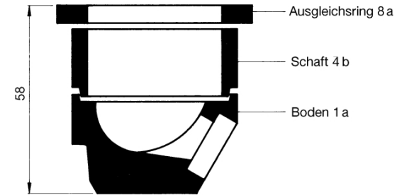
Schema Straßeneinlauf
